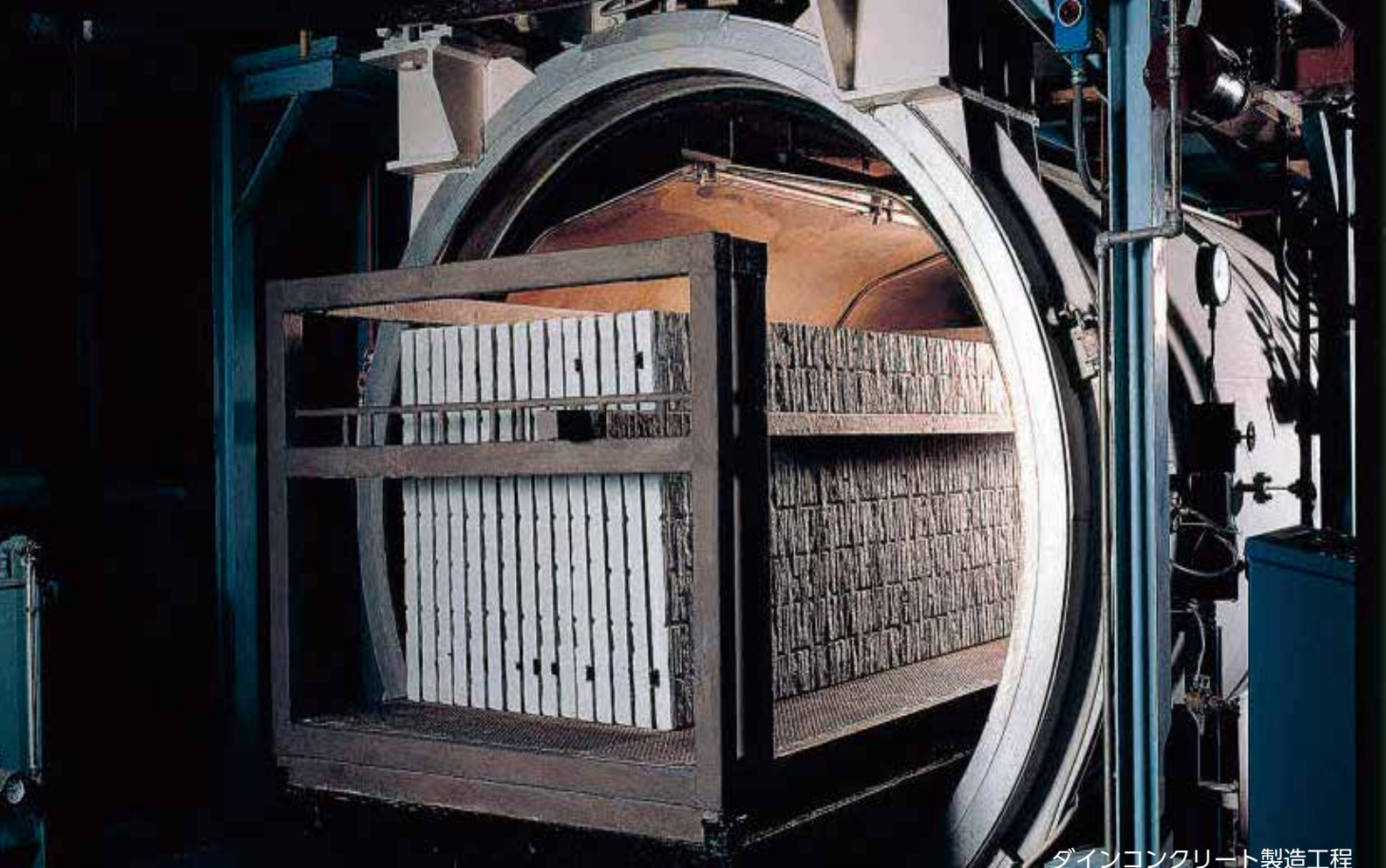
ダイコンクリート製造工程
