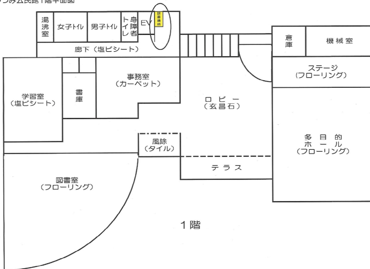
古河市つつみ公民館1階平面図
