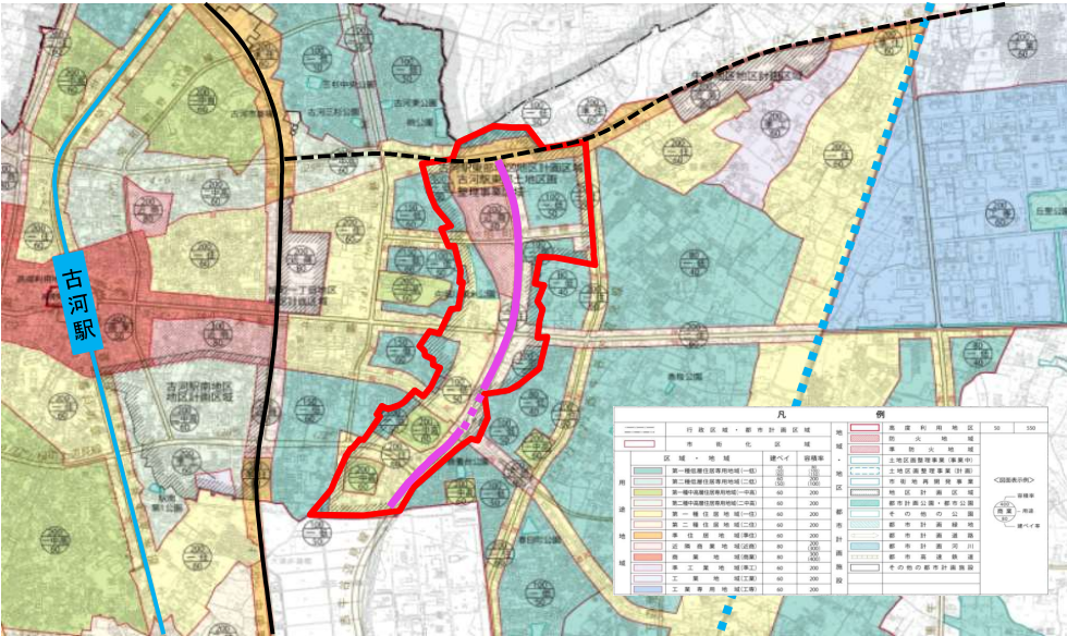
古河駅都市計画事業 古河駅東部土地区画整理事業 位置図
