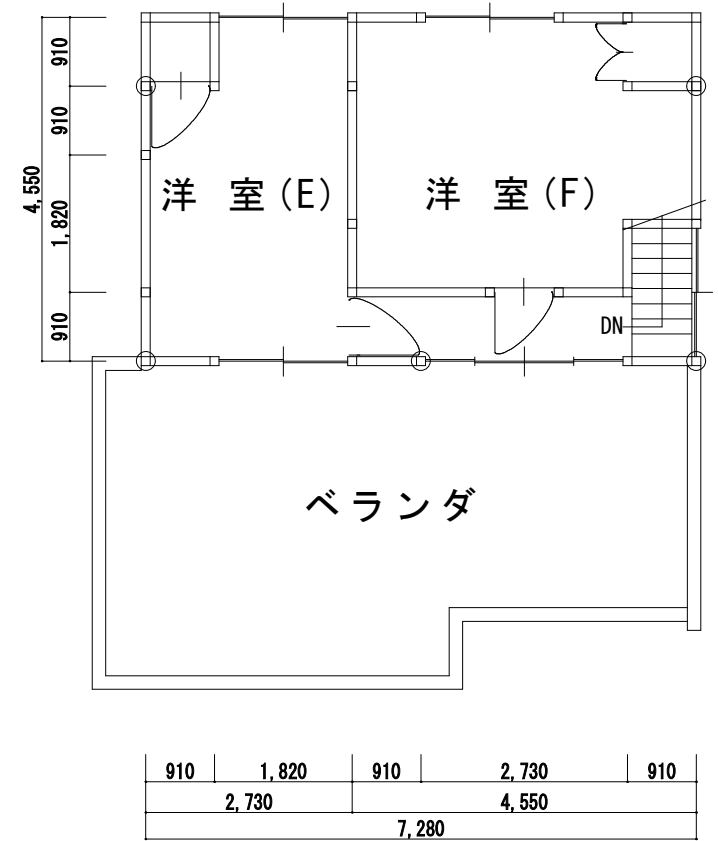
2階平面図
