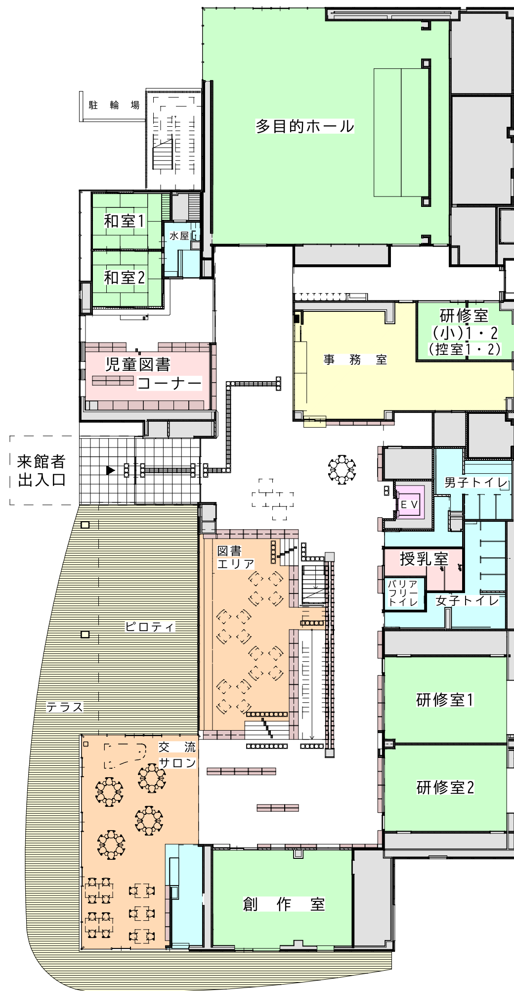
1 階平面図
