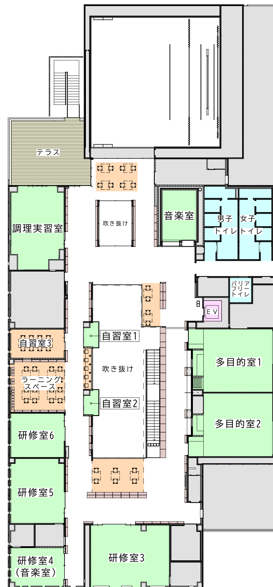
2 階平面図
