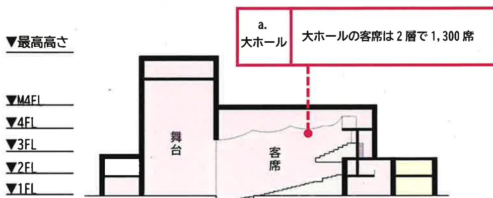
図 4.10 断面イメージ
