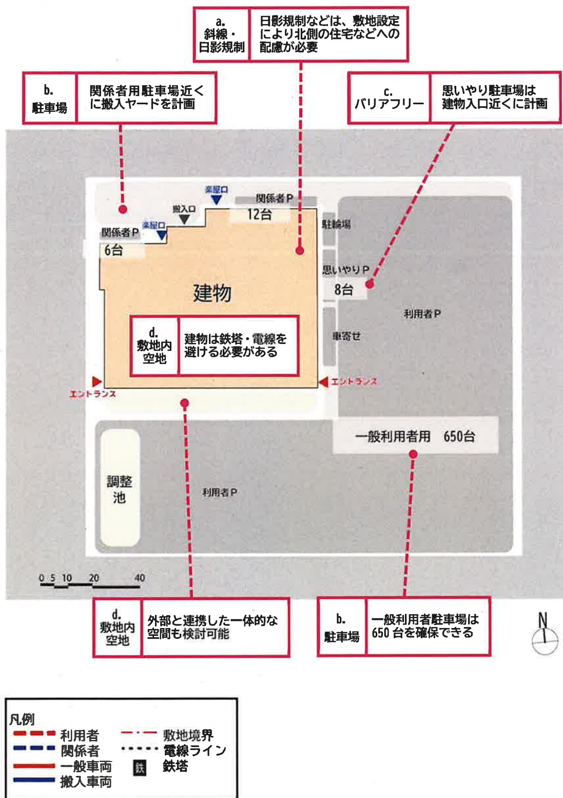
図 4.6 配置検討結果の詳細イメージ
