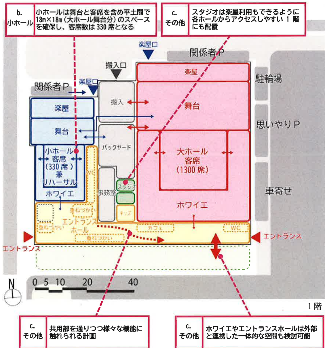
図 4.8 平面イメージ (1/2)
