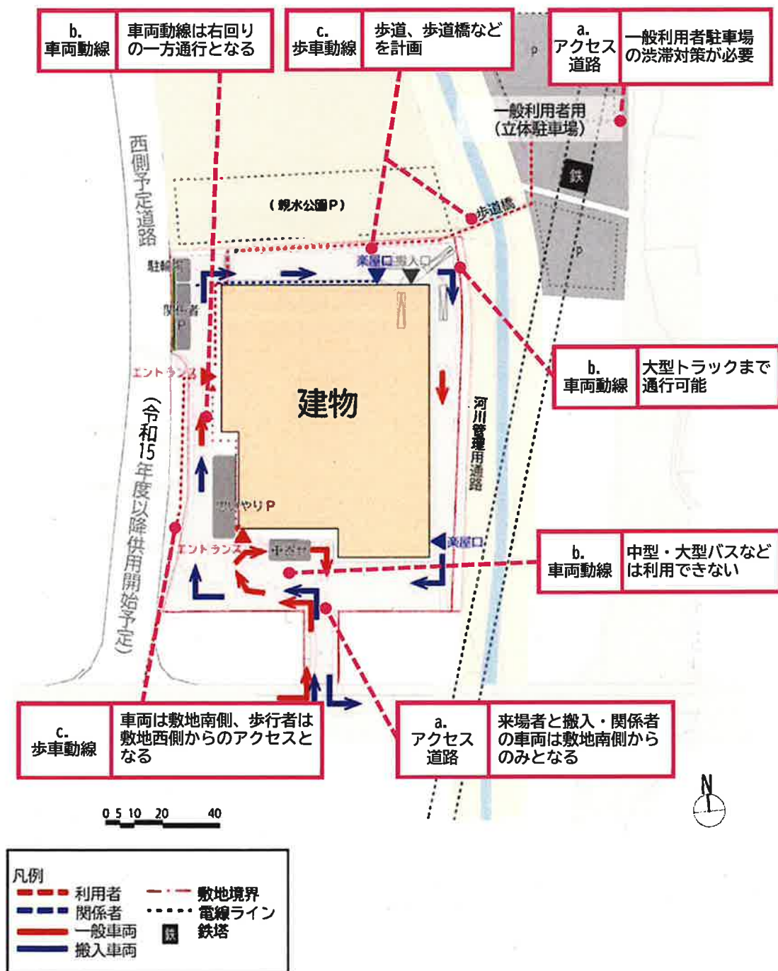
図 4.2 動線検討結果の詳細イメージ
